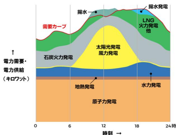
図 32：電力の需要と供給のバランス
