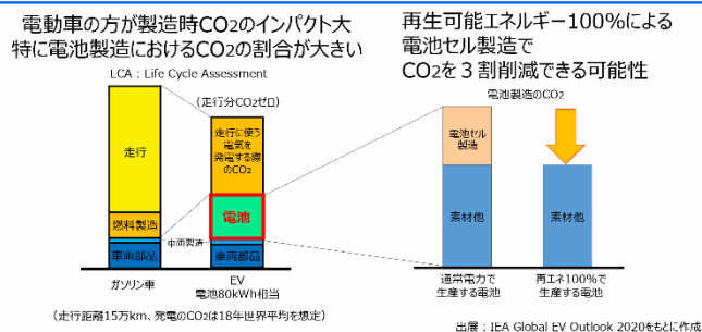
図 40：ガソリン車と電気自動車の LCA 評価
