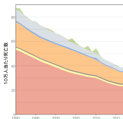
図 61：気候に関連する死亡数の推移
