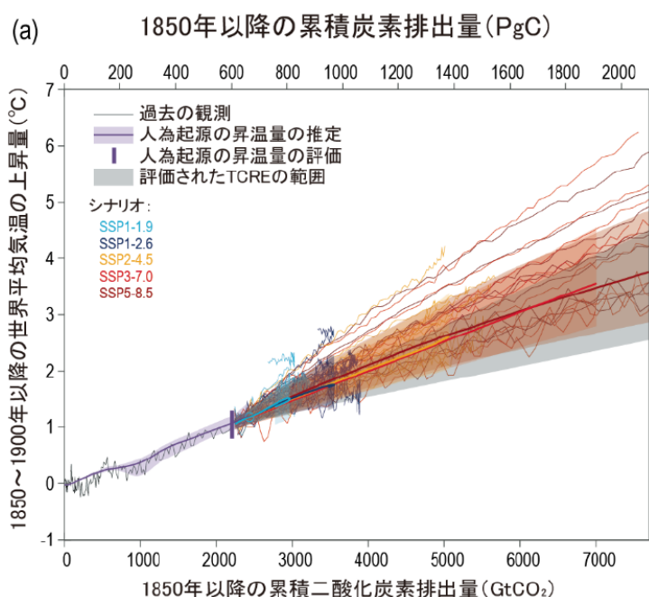
図 66：傾きを TCRE とする累積 CO 2 排出量と気温上昇の比例関係
