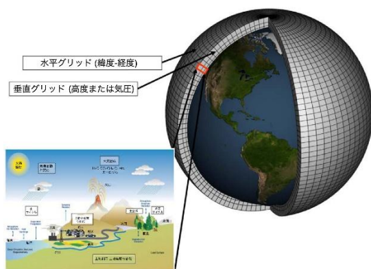
図 63：地球気候モデルの概念図
