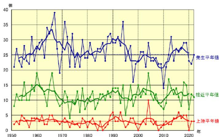
図 56：台風の発生数、日本への接近数・上陸数の経年変化
