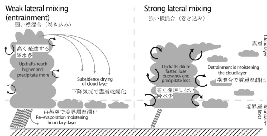
図 64：雲の対流に関する「巻き込み」のパラメーターの効果
