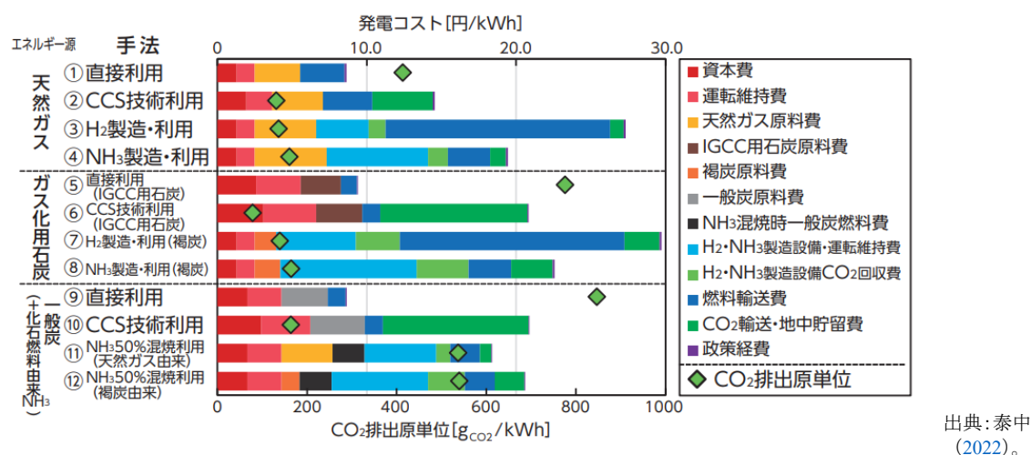
図 42：脱炭素技術と発電コスト
