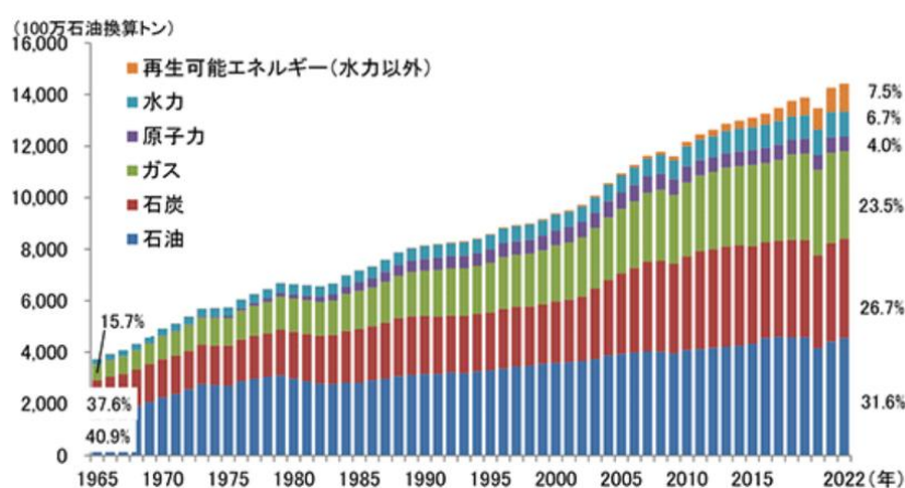
図 43：世界のエネルギー消費量の推移
