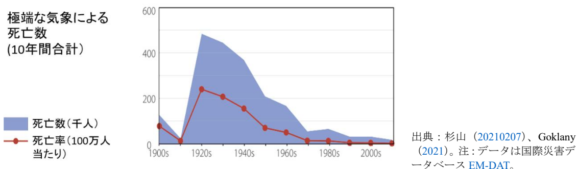
図 60：世界全体の極端な気象による死亡数の推移
