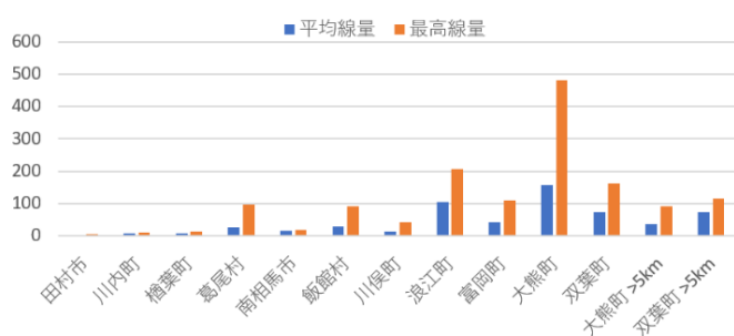
図 20：避難指示市町村の最初の 1 年間の線量
