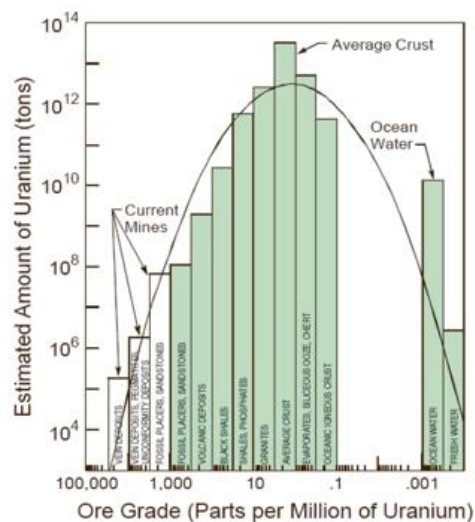
図 25：地殻のウラン分布
