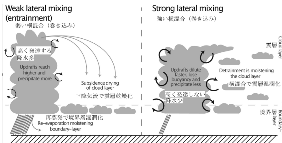
図 63：雲の対流に関する「巻き込み」のパラメーターの効果
